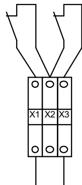
CABLAGE CONTACT NC
