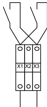
CABLAGE CONTACT NO
