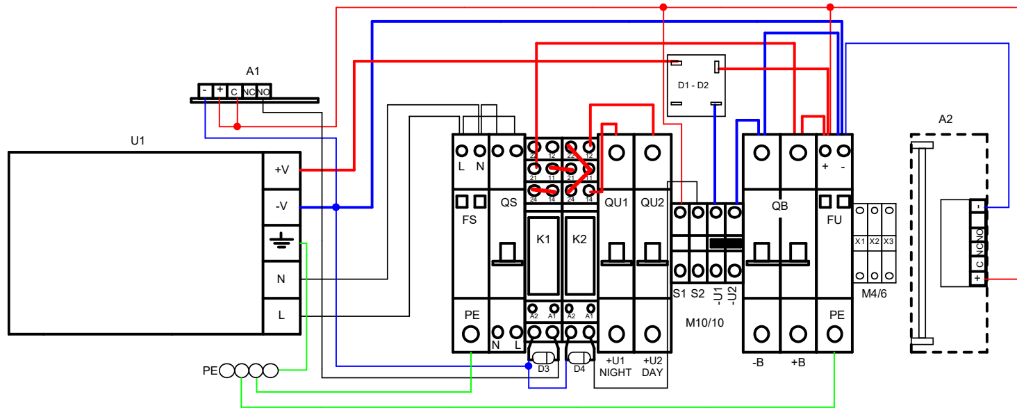
CABLAGE CONTACT NC
