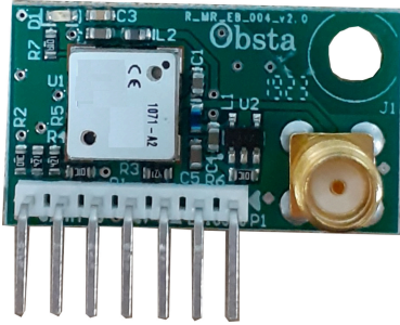
GPS PCB
