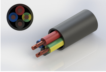
cable 4G1,5
